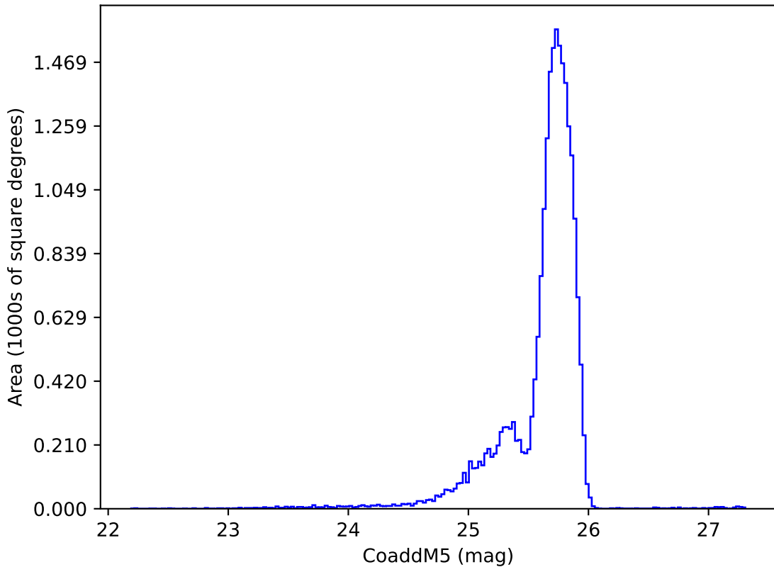
retro_baseline_v2.0_10yrs u: CoaddM5
