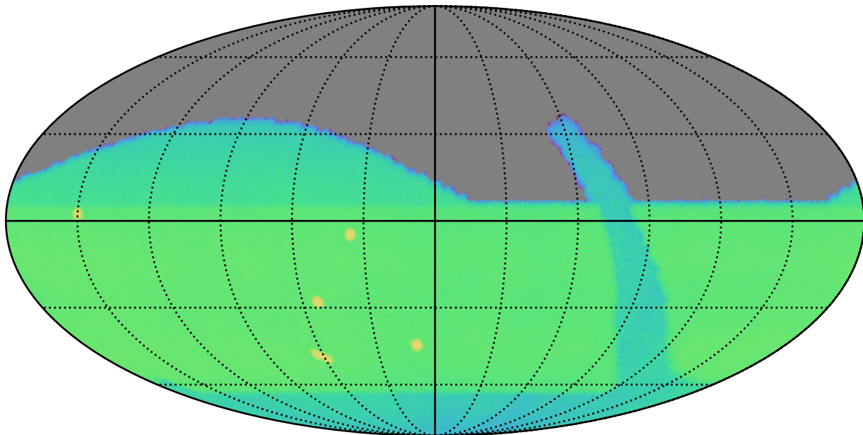
retro_baseline_v2.0_10yrs i: CoaddM5
