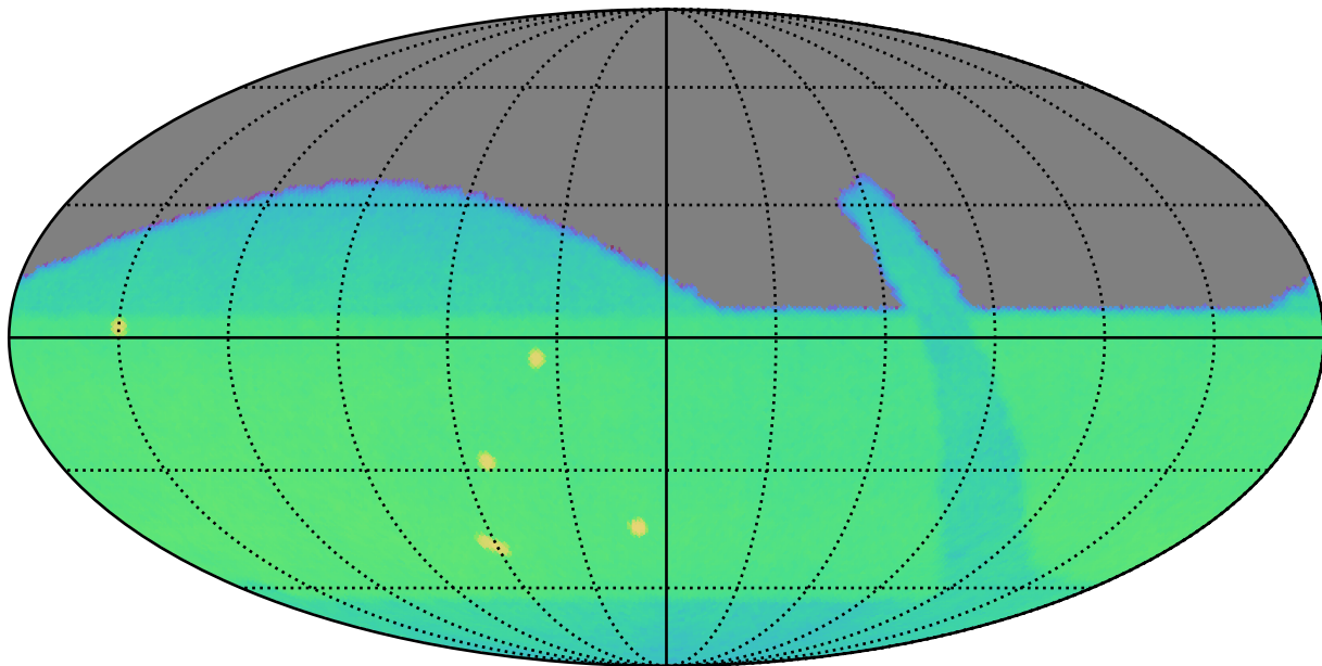
retro_baseline_v2.0_10yrs g: CoaddM5
