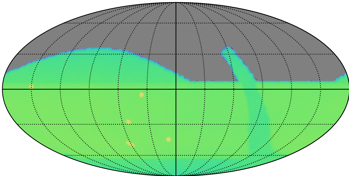
retro_baseline_v2.0_10yrs : CoaddM5
