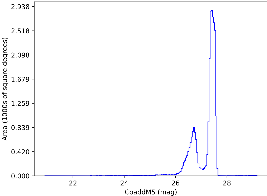
retro_baseline_v2.0_10yrs : CoaddM5
