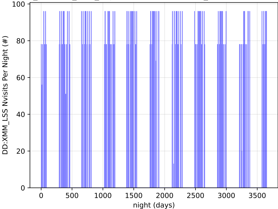
retro_baseline_v2.0_10yrs all bands: DD:XMM_LSS Nvisits Per Night
