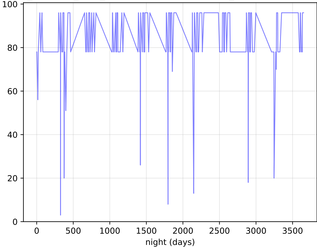
retro_baseline_v2.0_10yrs all bands: DD:XMM_LSS Nvisits Per Night
