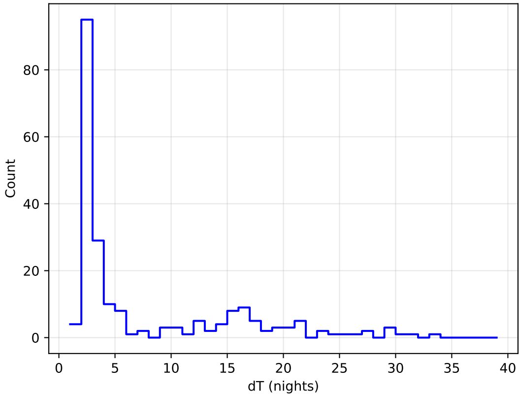
retro_baseline_v2.0_10yrs all bands: DD:ELAISS1 Delta Nights Histogram
