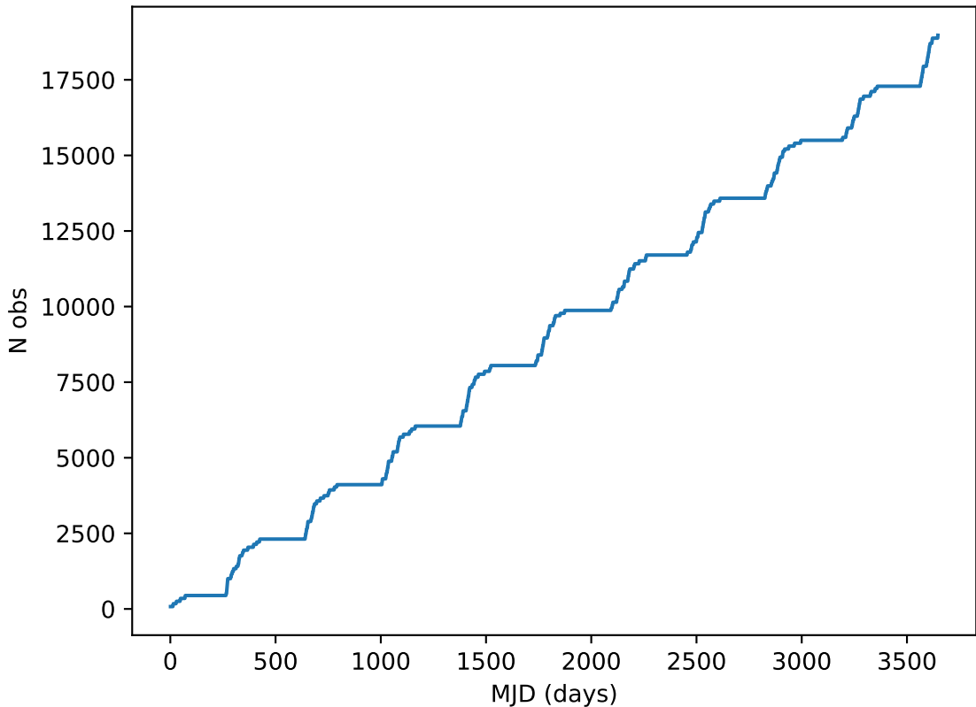
retro_baseline_v2.0_10yrs all bands: DD:ELAISS1 Cumulative NVisits
