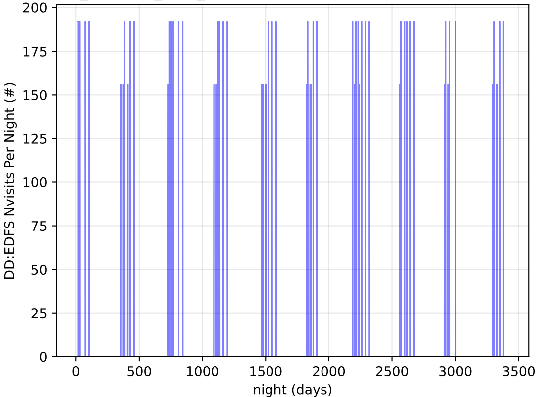
retro_baseline_v2.0_10yrs all bands: DD:EDFS Nvisits Per Night
