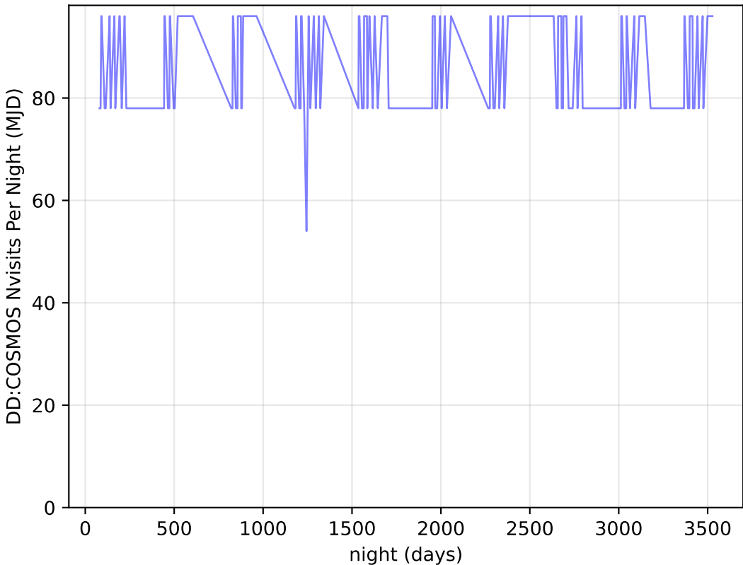
retro_baseline_v2.0_10yrs all bands: DD: COSMOS Nvisits Per Night
