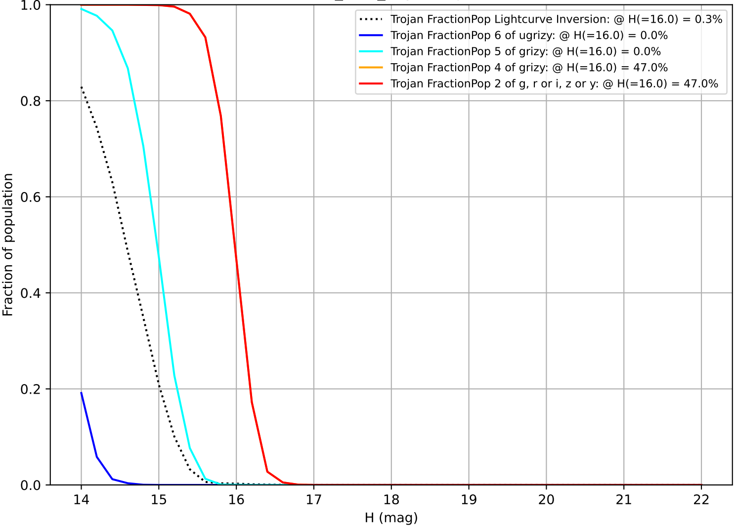
octo_v3.4_10yrs Trojan
