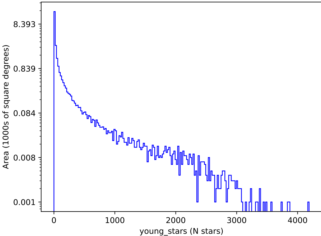
octo_v3.4_10yrs : young_stars
