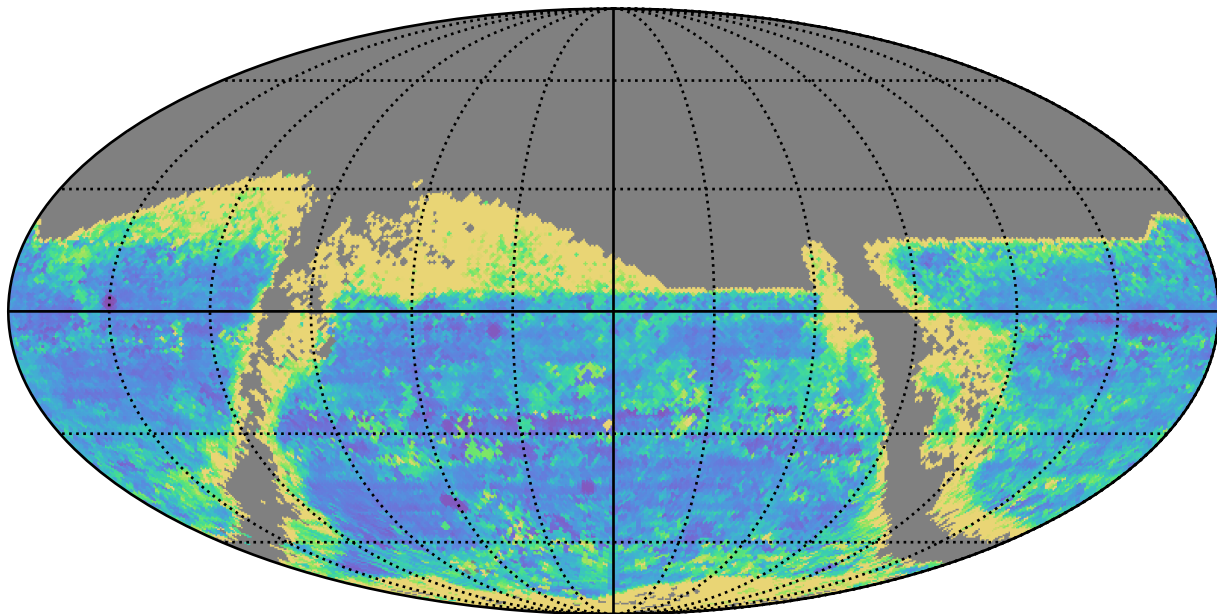
octo_v3.4_10yrs : TDC_precision
