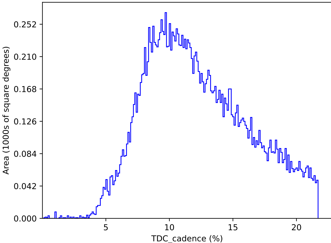
octo_v3.4_10yrs : TDC_cadence
