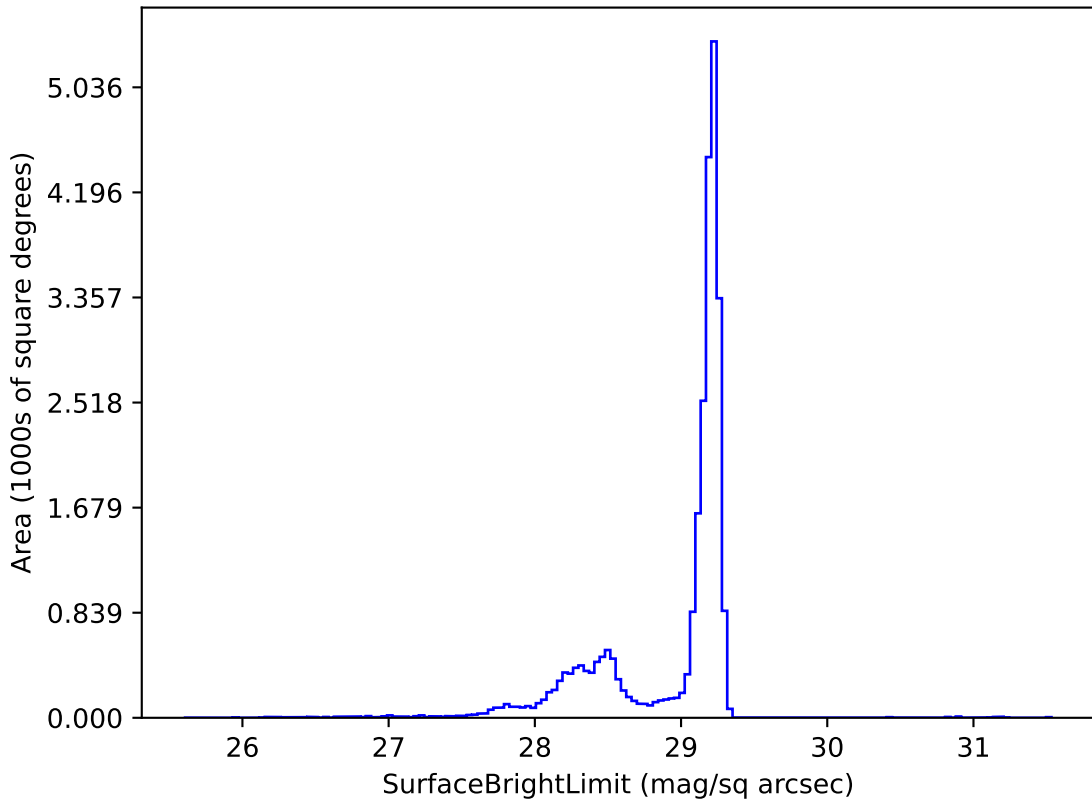
octo_v3.4_10yrs z: SurfaceBrightLimit
