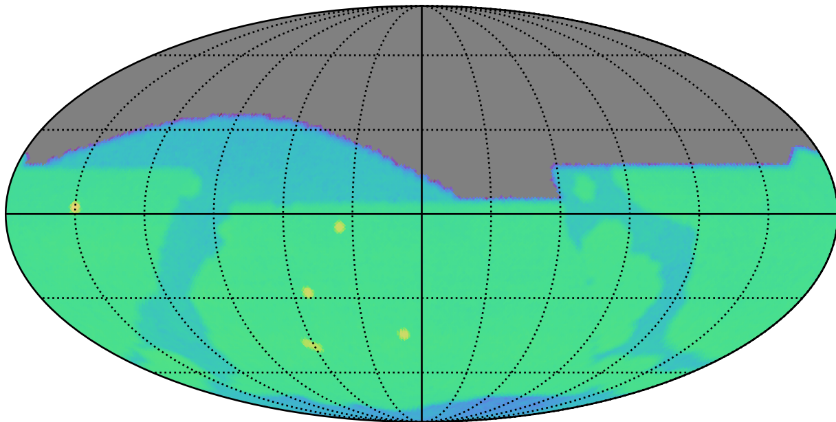
octo_v3.4_10yrs r: SurfaceBrightLimit
