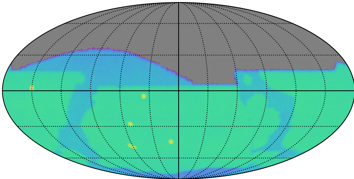
octo_v3.4_10yrs i: SurfaceBrightLimit
