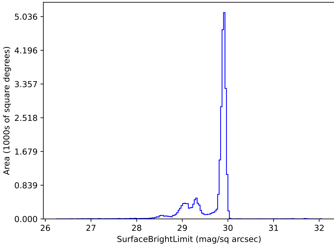
octo_v3.4_10yrs i: SurfaceBrightLimit
