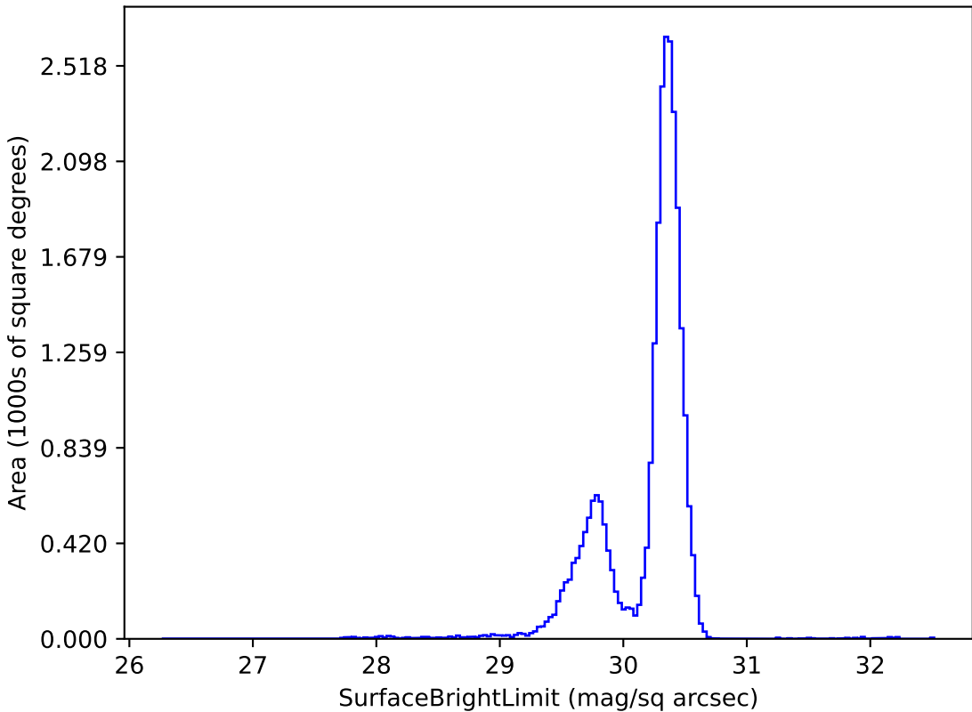
octo_v3.4_10yrs g: SurfaceBrightLimit
