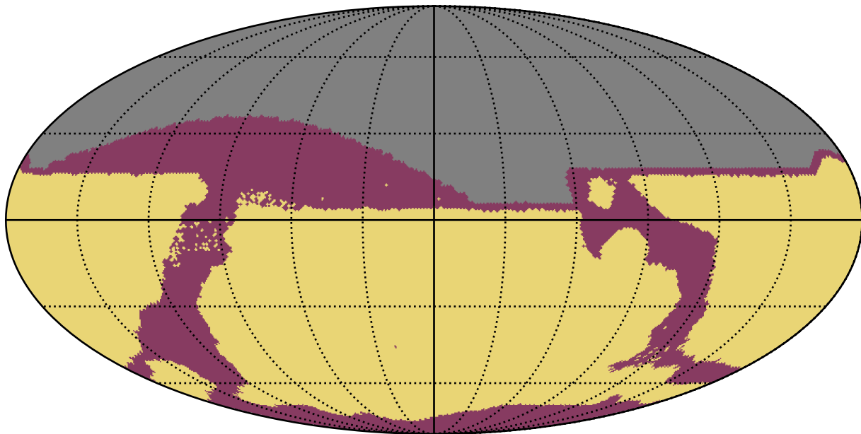
octo_v3.4_10yrs : RapidRevisits
