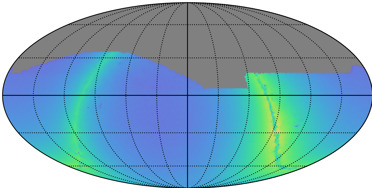
octo_v3.4_10yrs z: Nstars_no_crowding
