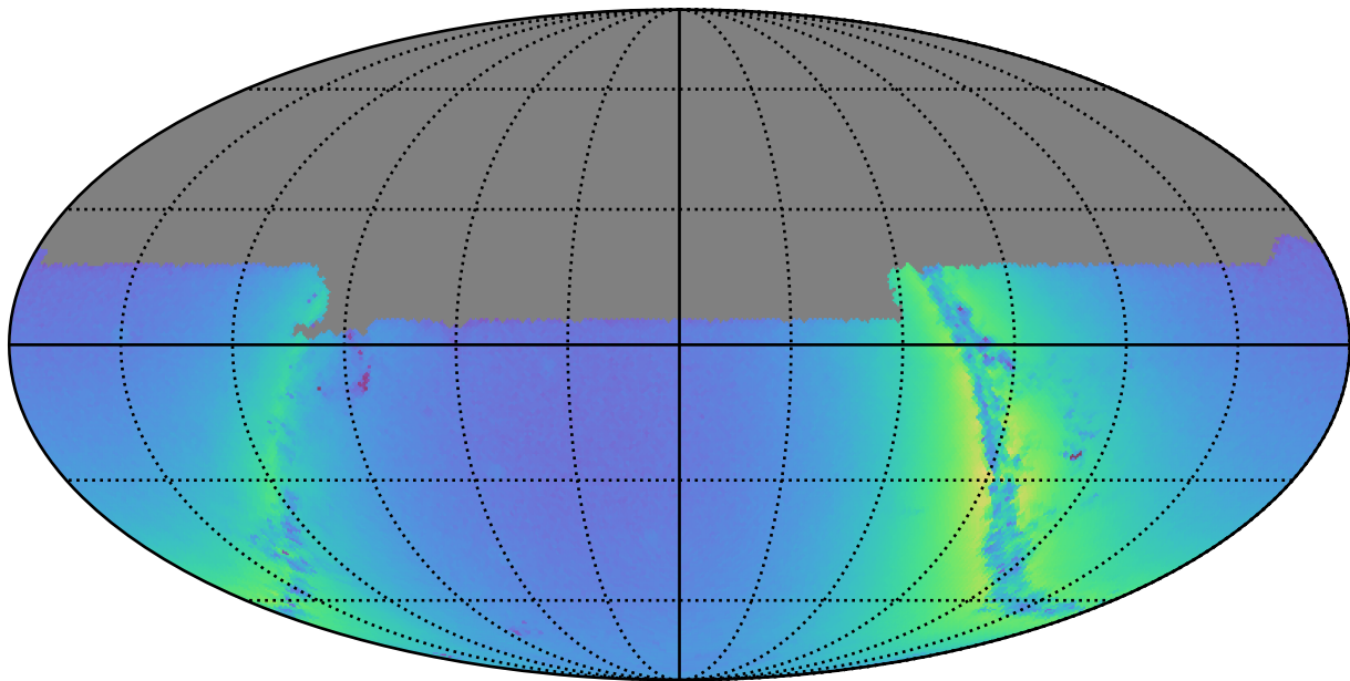
octo_v3.4_10yrs u: Nstars_no_crowding
