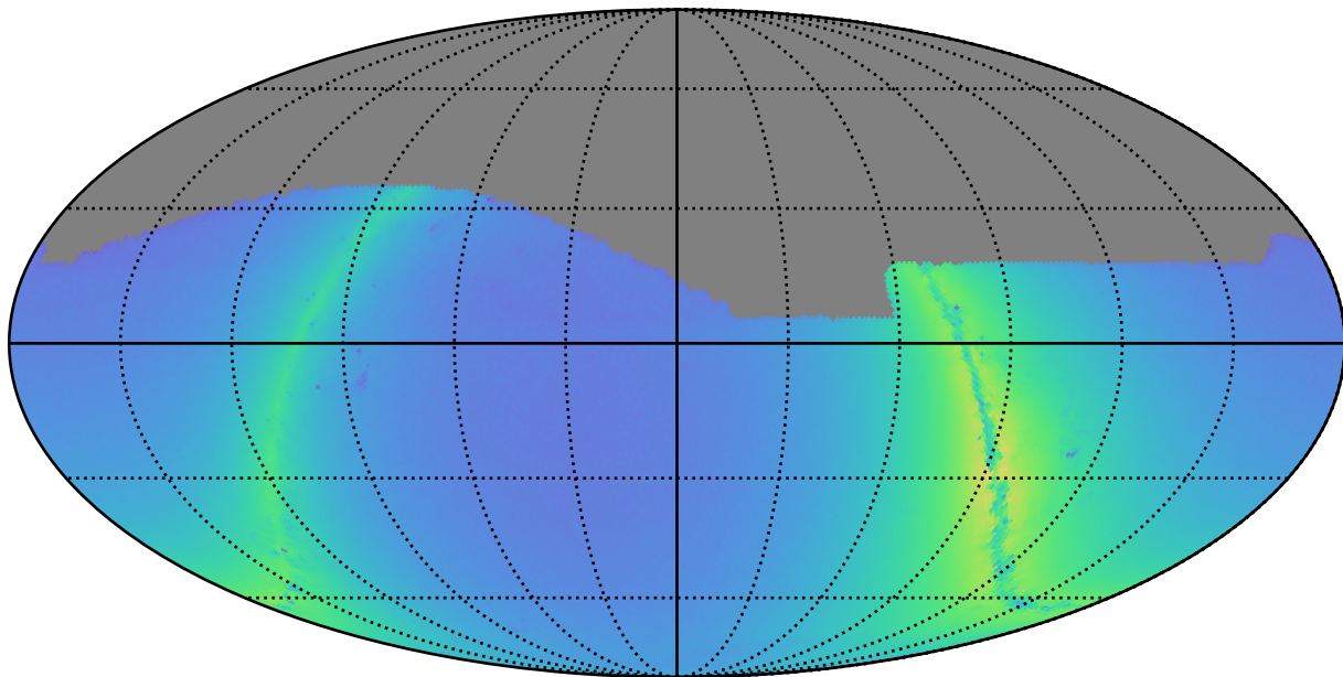
octo_v3.4_10yrs i: Nstars_no_crowding
