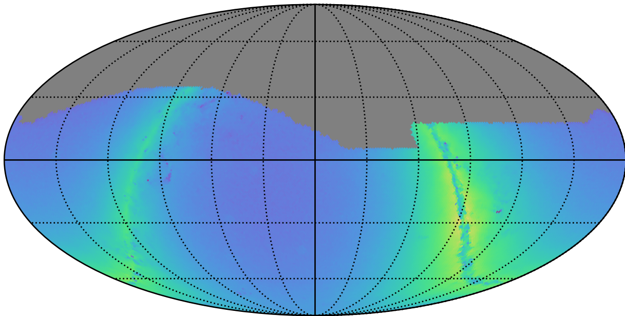
octo_v3.4_10yrs g: Nstars_no_crowding
