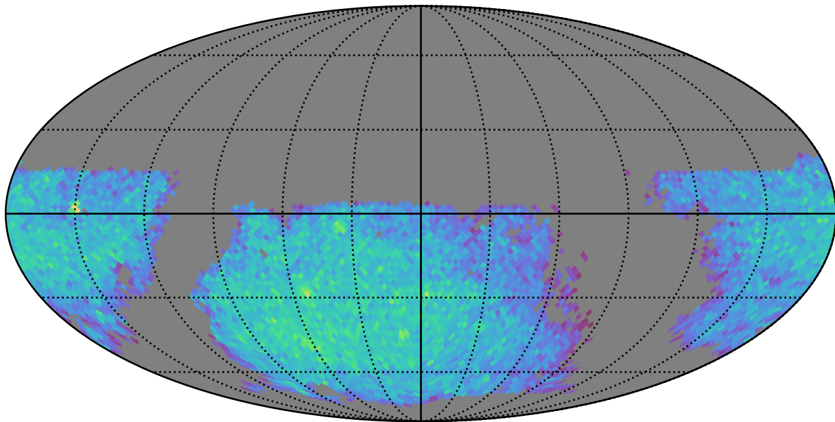
octo_v3.4_10yrs gi: LVDwarfs
