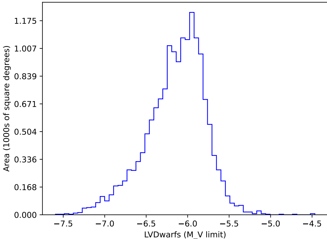
octo_v3.4_10yrs gi: LVDwarfs
