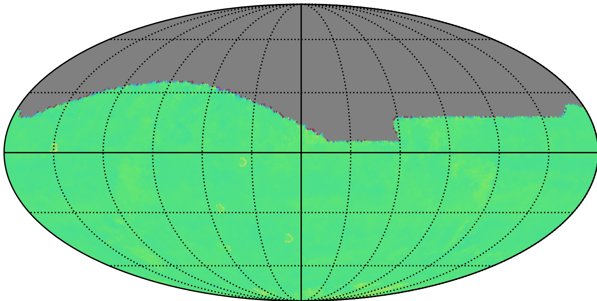
octo_v3.4_10yrs r: Kuiper rotTelPos
