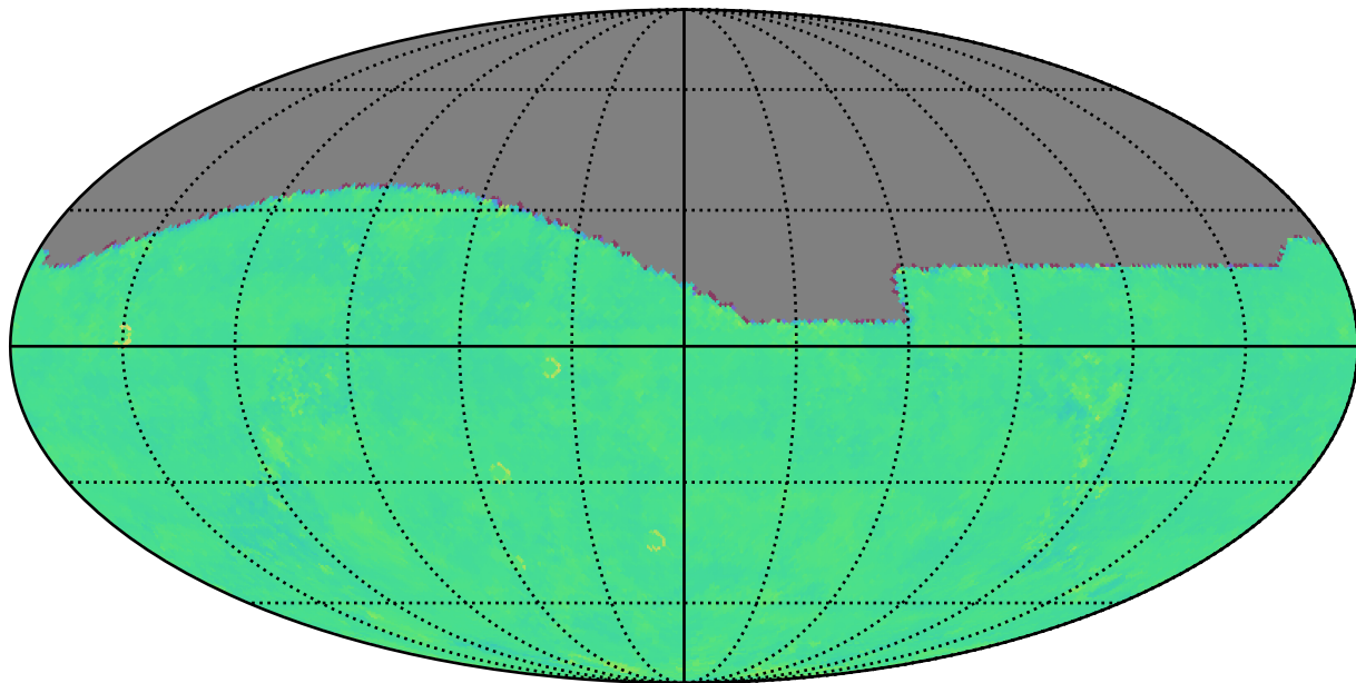
octo_v3.4_10yrs g: Kuiper rotTelPos
