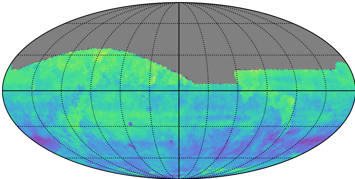
octo_v3.4_10yrs z: Kuiper rotSkyPos
