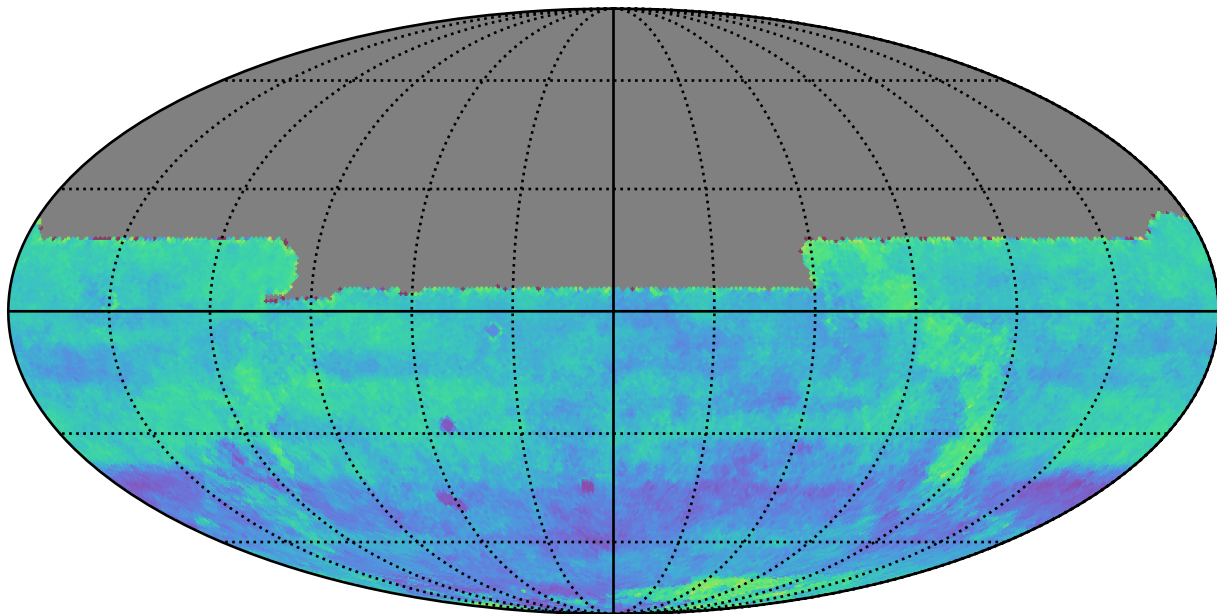
octo_v3.4_10yrs y: Kuiper rotSkyPos
