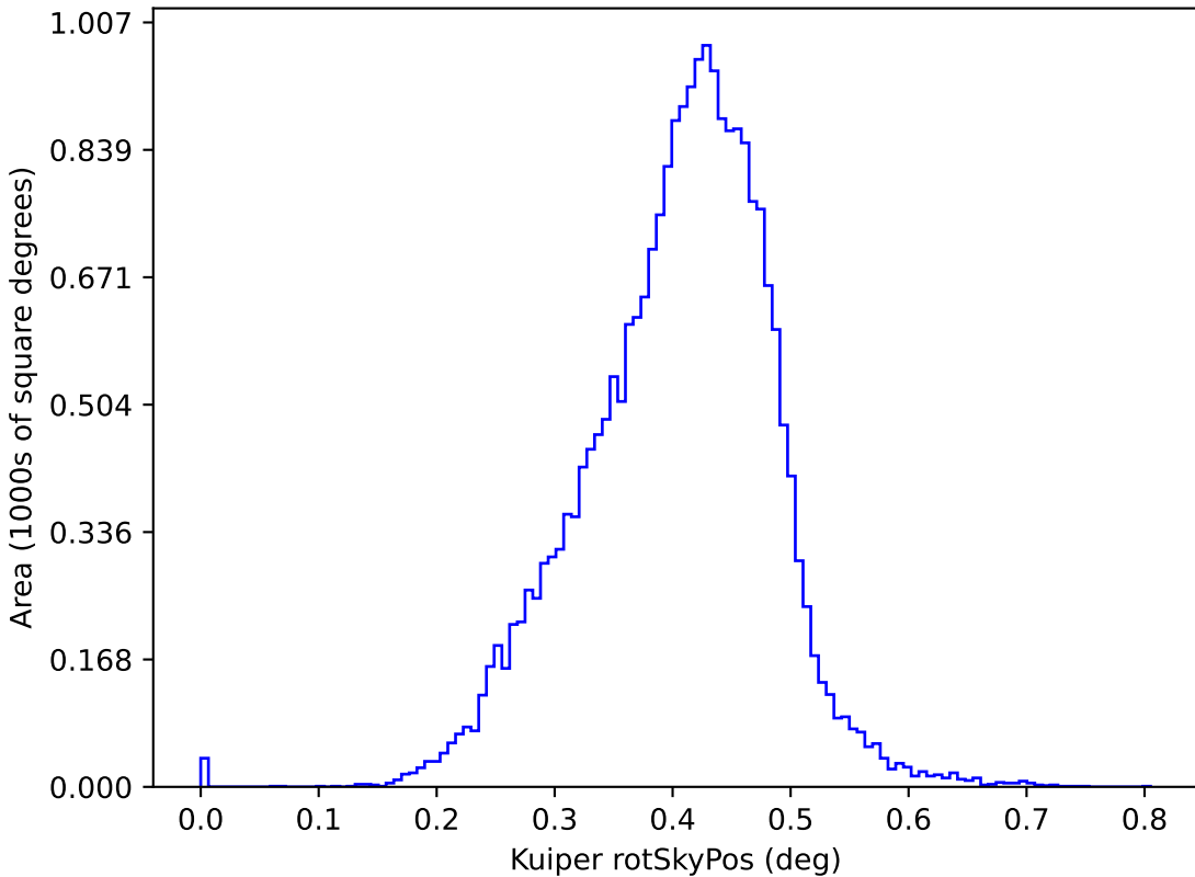
octo_v3.4_10yrs y: Kuiper rotSkyPos
