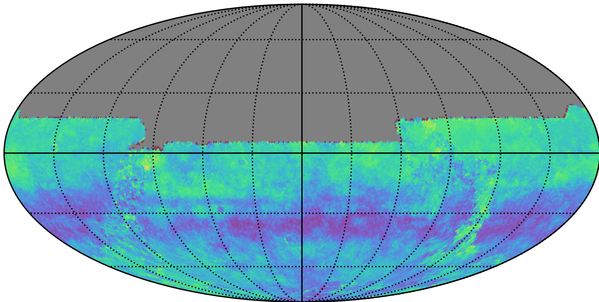
octo_v3.4_10yrs u: Kuiper rotSkyPos
