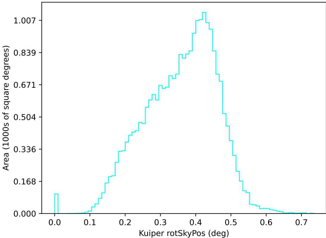
octo_v3.4_10yrs u: Kuiper rotSkyPos
