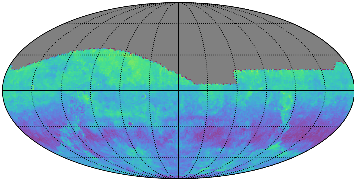
octo_v3.4_10yrs g: Kuiper rotSkyPos
