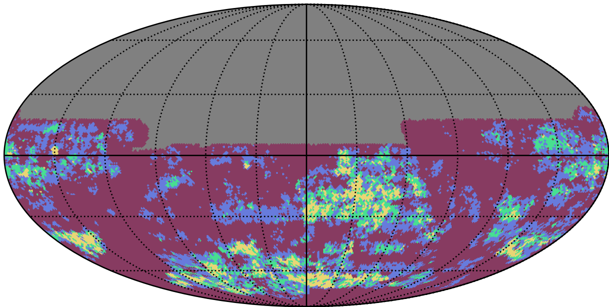
octo_v3.4_10yrs y band: Gaps_7hr
