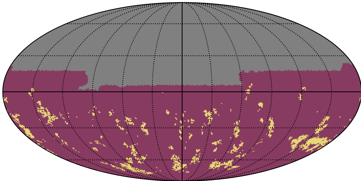
octo_v3.4_10yrs u band: Gaps_7hr
