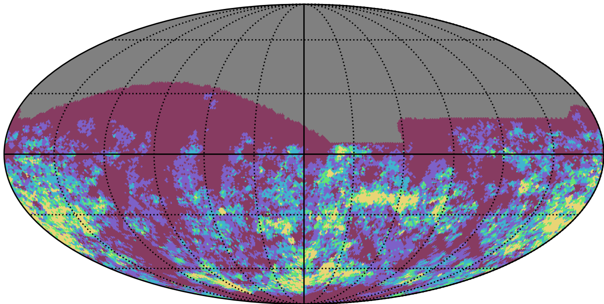
octo_v3.4_10yrs i band: Gaps_7hr
