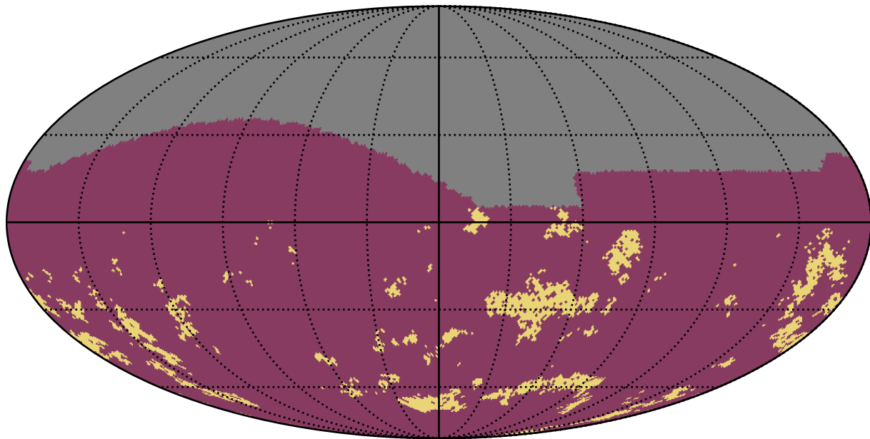
octo_v3.4_10yrs g band: Gaps_7hr
