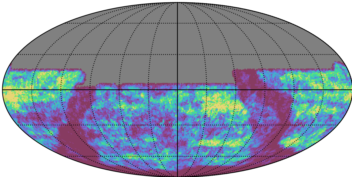
octo_v3.4_10yrs y band: Gaps_3hr
