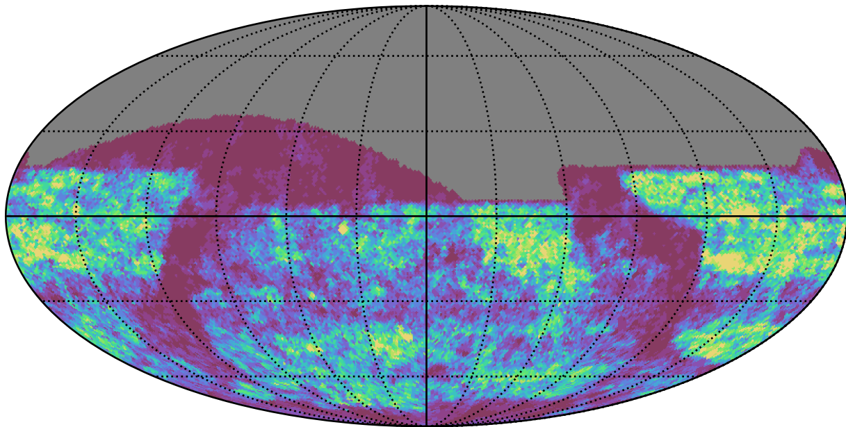
octo_v3.4_10yrs i band: Gaps_3hr
