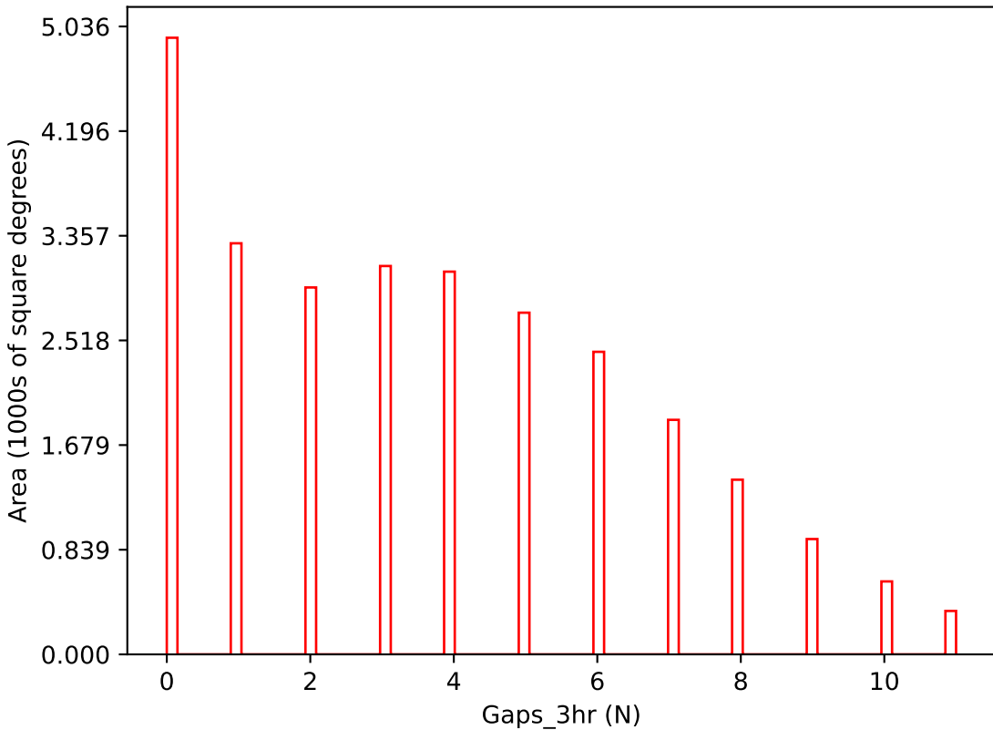
octo_v3.4_10yrs i band: Gaps_3hr
