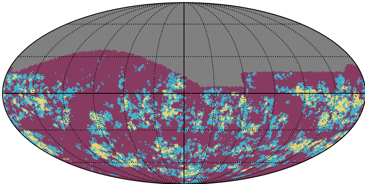
octo_v3.4_10yrs g band: Gaps_3hr
