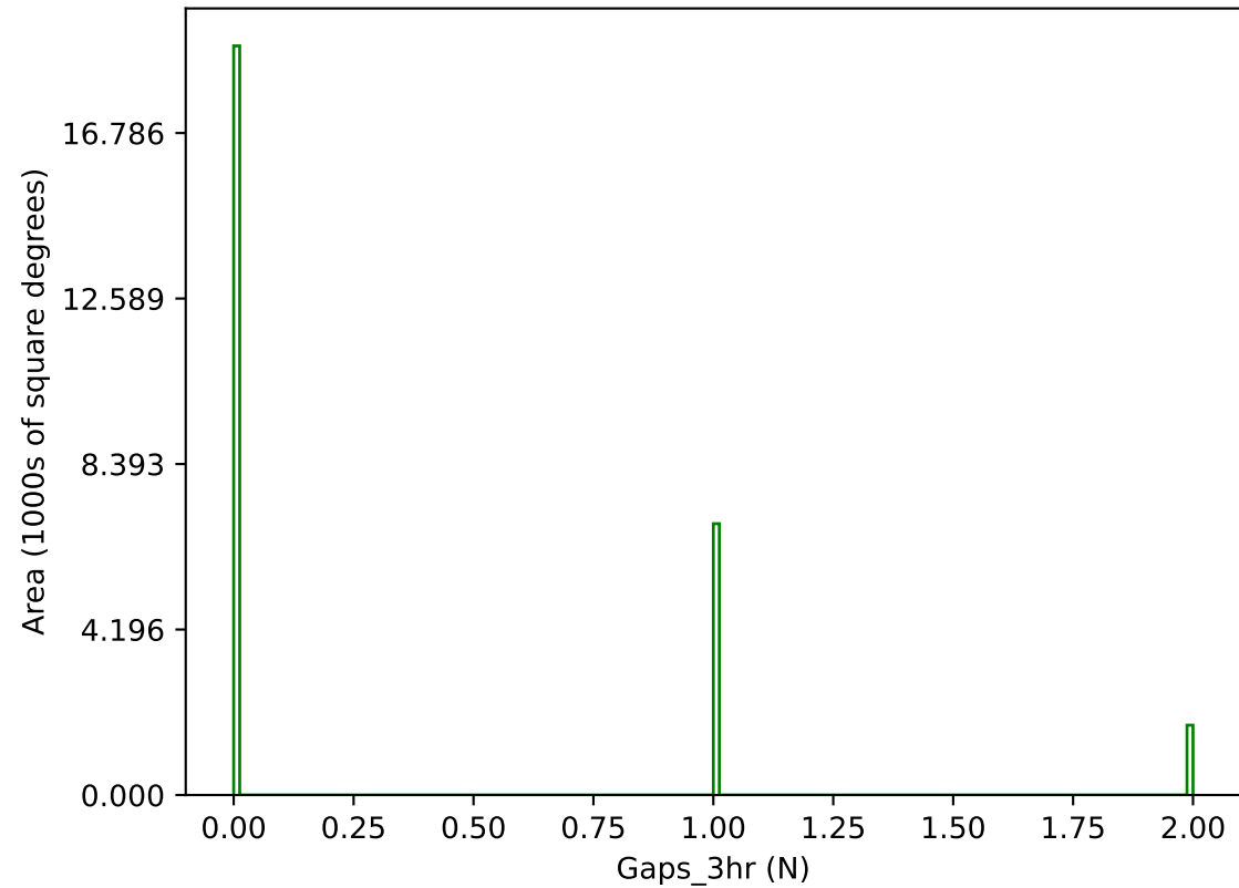
octo_v3.4_10yrs g band: Gaps_3hr
