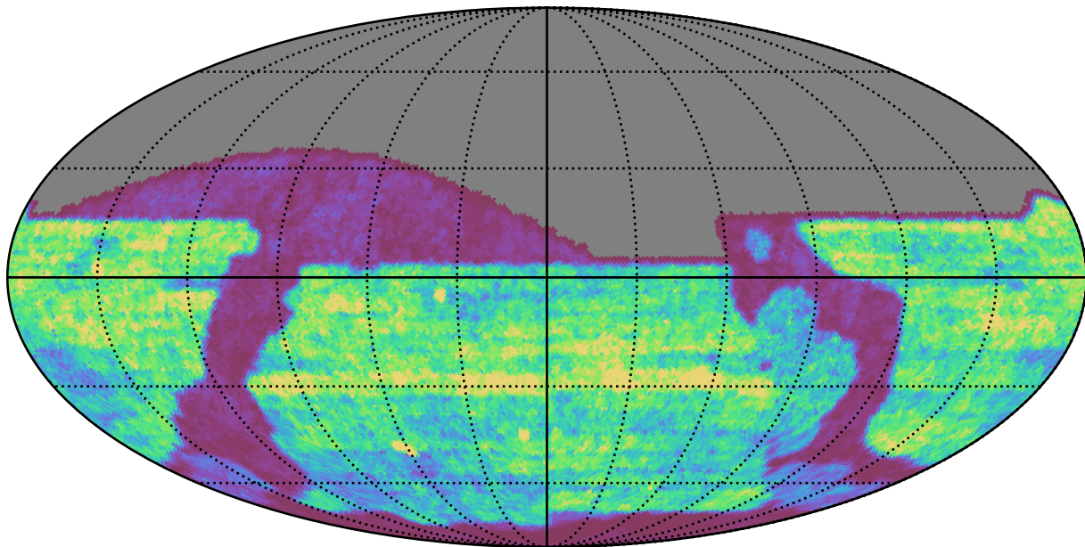
octo_v3.4_10yrs r band: Gaps_24hr
