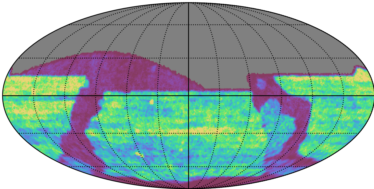
octo_v3.4_10yrs i band: Gaps_24hr
