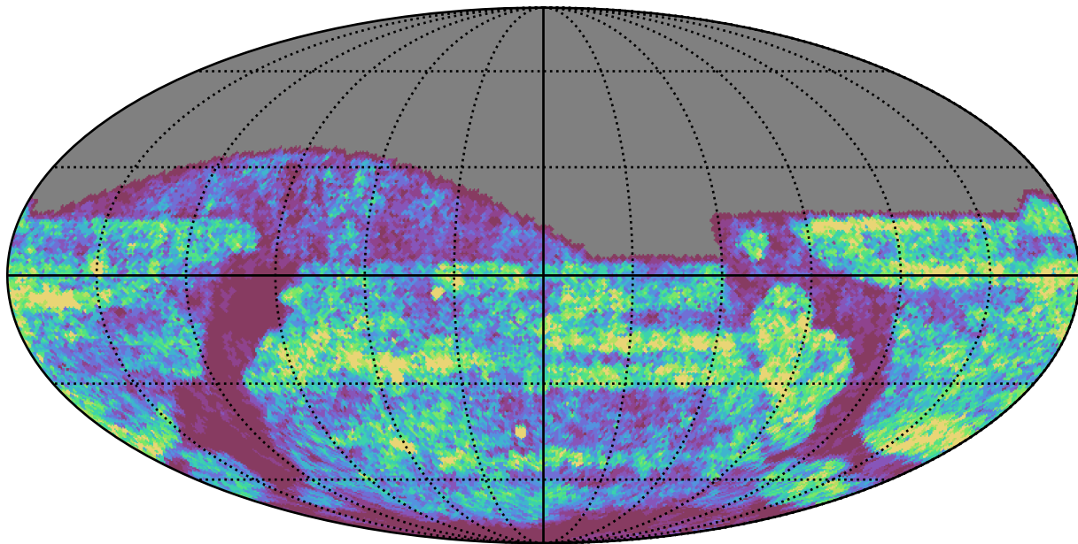
octo_v3.4_10yrs g band: Gaps_24hr
