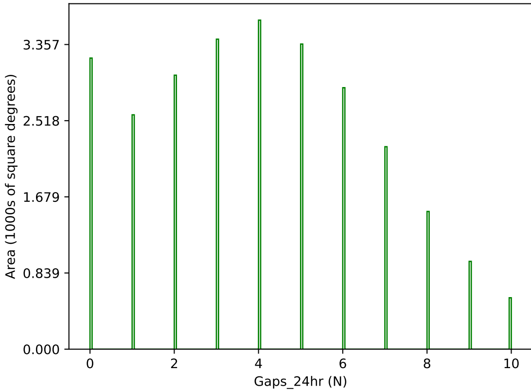
octo_v3.4_10yrs g band: Gaps_24hr
