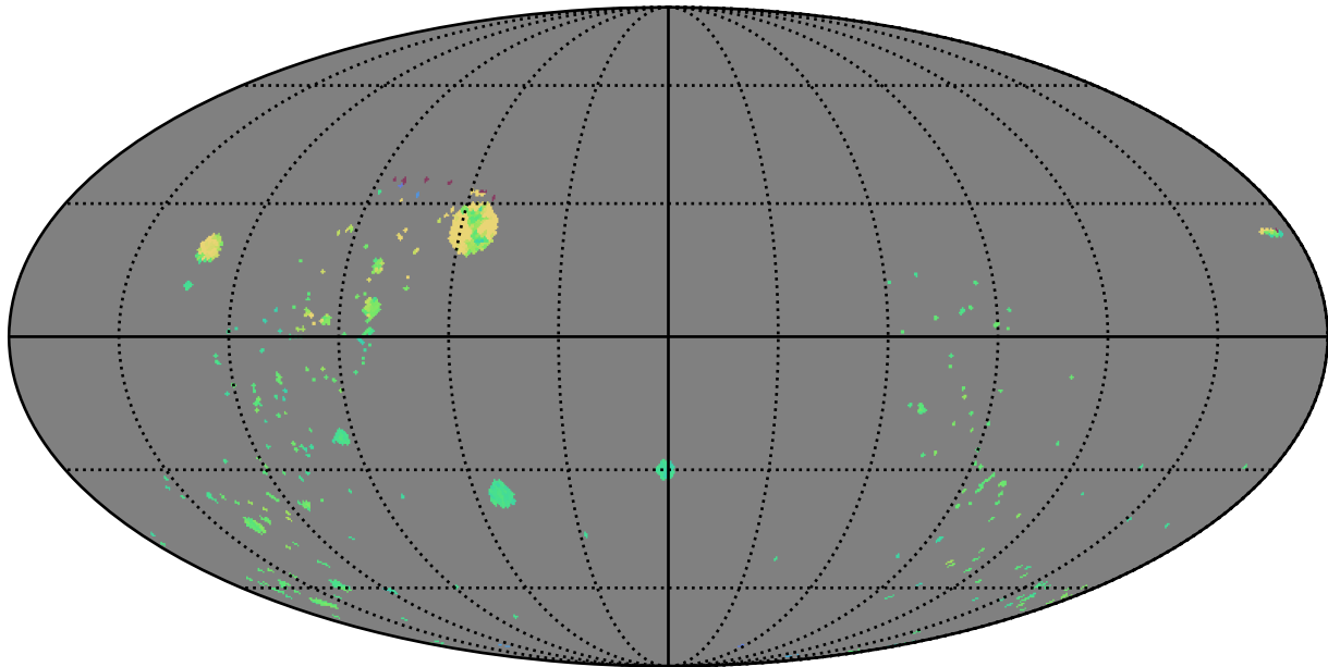
octo_v3.4_10yrs : GalplaneTimePerFilter_open_clusters_map_i
