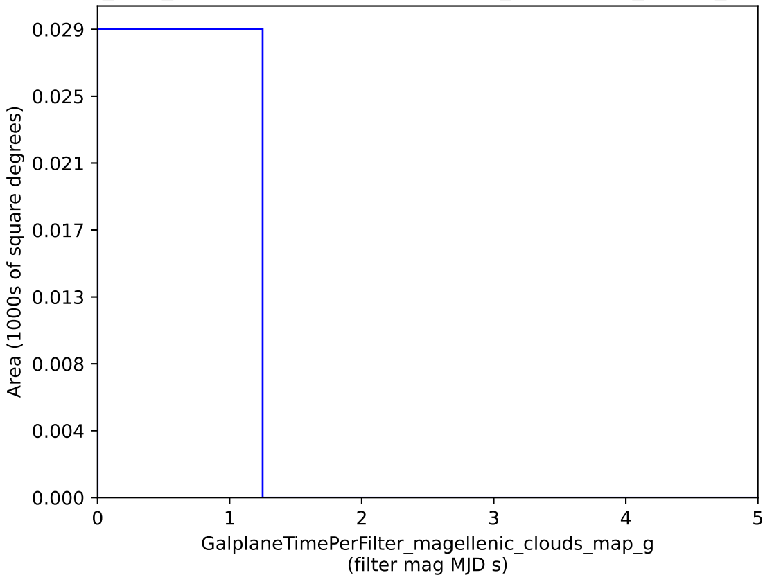
octo_v3.4_10yrs : GalplaneTimePerFilter_magellenic_clouds_map_g
