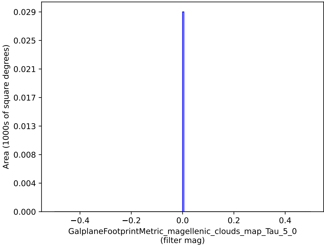
octo_v3.4_10yrs : GalplaneFootprintMetric_magellanic_clouds_map_Tau_5_0
